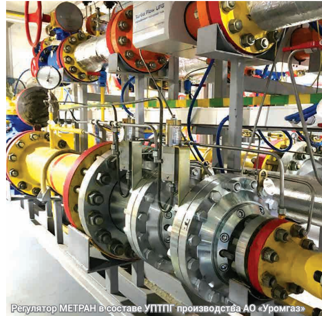
Регулятор МЕТРАН в составе УПТПГ производства АО «Уромгаз»
