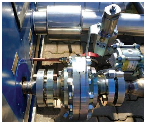
Блок подготовки АГМБ для ГПА ООО «Газхолдтехника»
