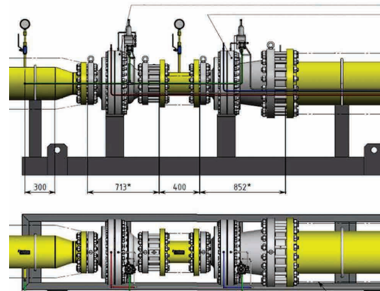
Пример импульсной обвязки
