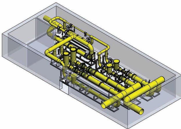
Пример визуализации ГРП в 3D
